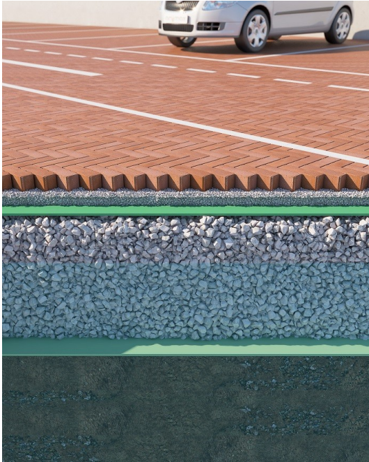
Drainatze jasangarriko sistemaren geruzak
